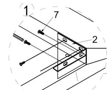
ヘッドボードとフットボードを サイドフレームに取り付ける
